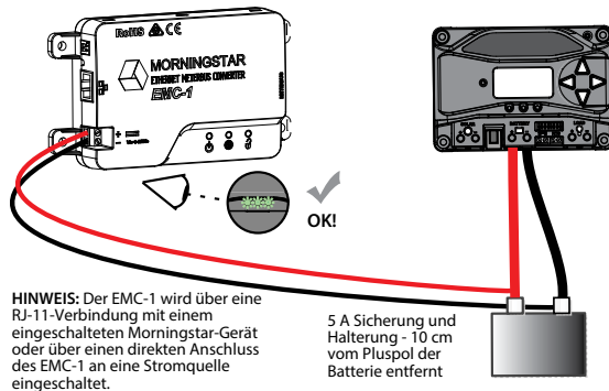
Abbildung 2-4. Anschluss an Spannungsversorgungsleitungen
