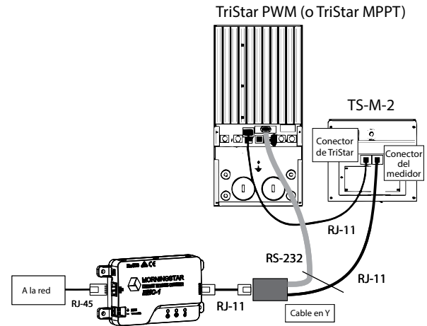
Figura 2-2. Recorrido del cable EMC-TS-M-2
