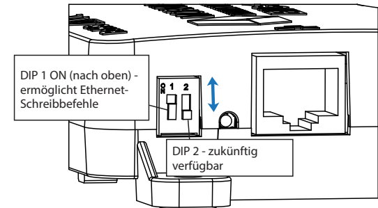
Abbildung 2-3. Funktionen der DIP-Schalter
