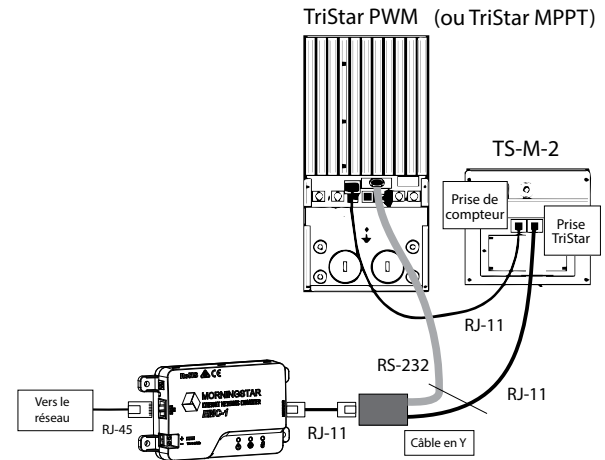
Figure 2-2. Acheminement des câbles EMC-TS-M-2
