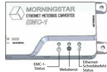
Abbildung 3-1. LED-Anzeigen
