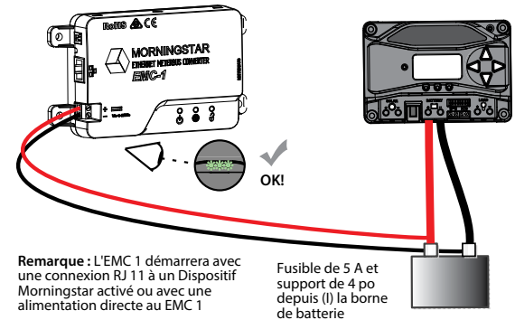
Figure 2-4. Connexion des câbles d'alimentation
